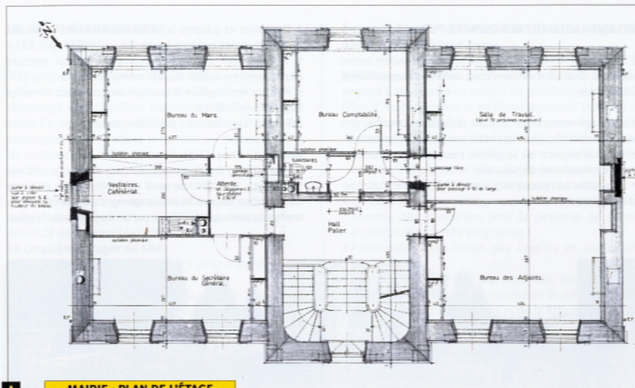
A MAIRIE : PLAN DE L'ÉTAGE
